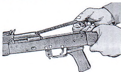
Вынимание возвратного механизма
